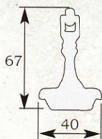
Réf.: DU 512 M
